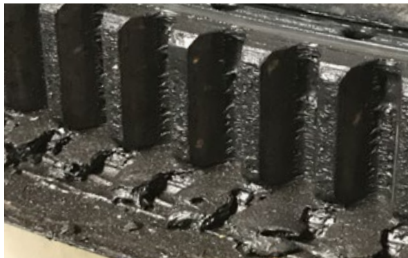
Reinigung Yaw-Verstellung
